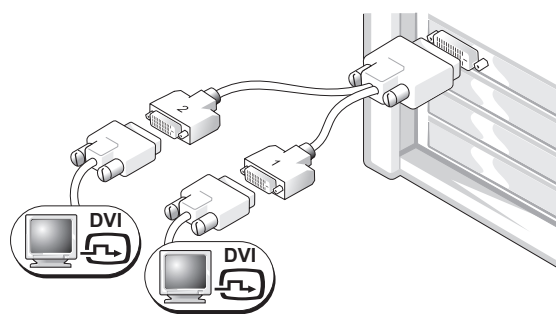
雙 DVI Y 形纜線配接器：
